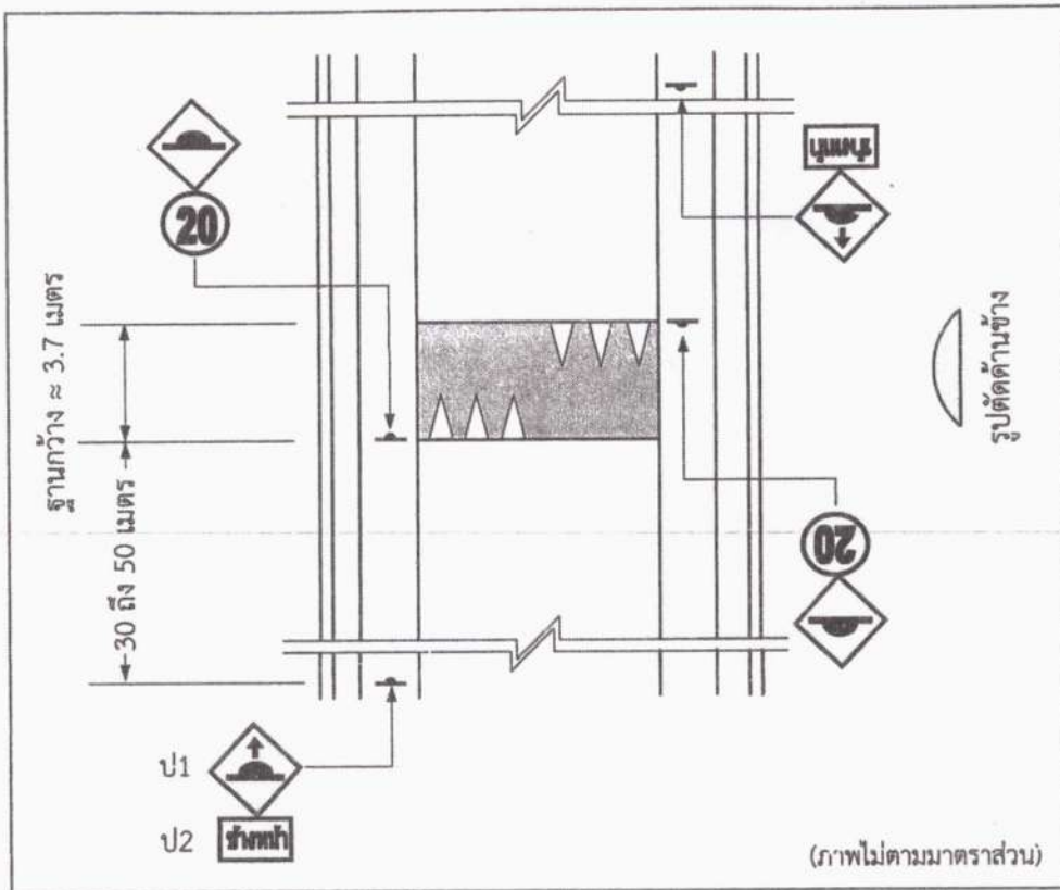
รูปที่ ๔ แบบแปลนการก่อสร้างเนินชะลอความเร็วแบบโค้งพาราโบลาในรูปแบบ Watts profile hump (ประยุกต์จาก AS ๑๗๔๒.๑๓-๒๐๐๙)
