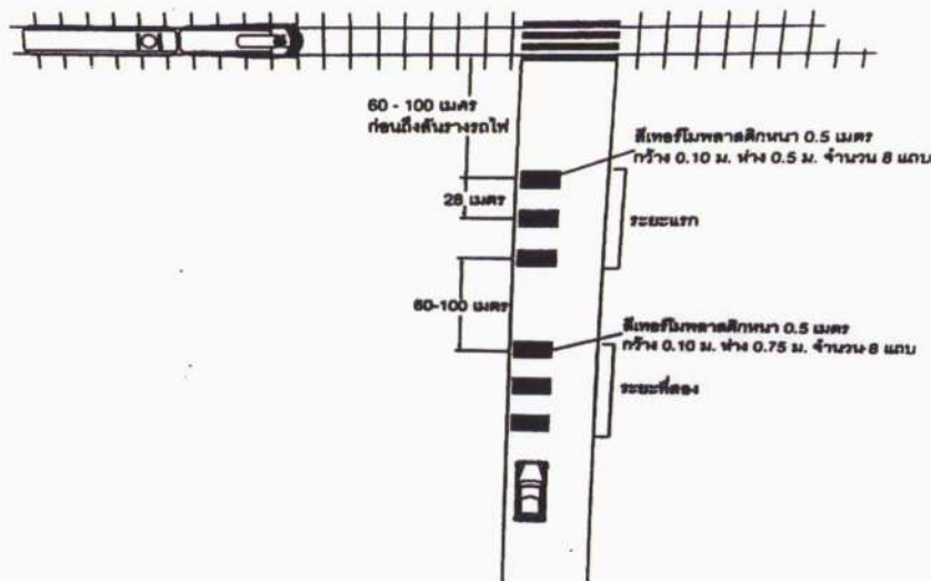
รูปที่ ๕๔ ตัวอย่างการติดตั้งรั้วเป็นสะดือที่บริเวณทางตัดผ่านทางรถไฟ
