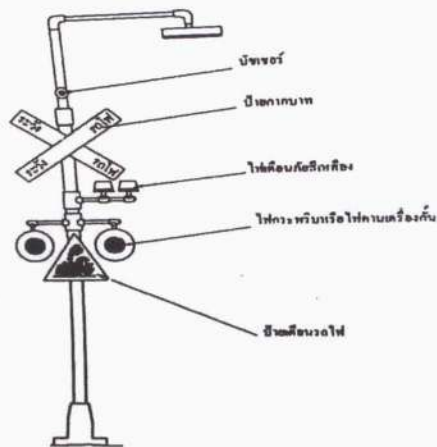
รูปที่ ๖๓ การติดตั้งสัญญาณไฟวามในกรณีที่ทางตัดผ่านติดตั้งเครื่องกั้นประเภทยัตโนมัต
